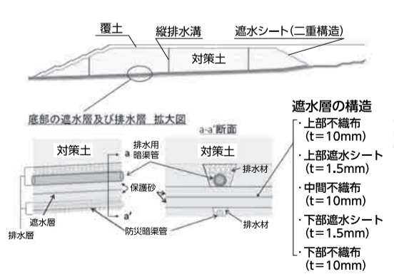
二重遮水シートによる封じ込め工法の詳細イメージ —第11回有識者会議JR東海提供資料より—
