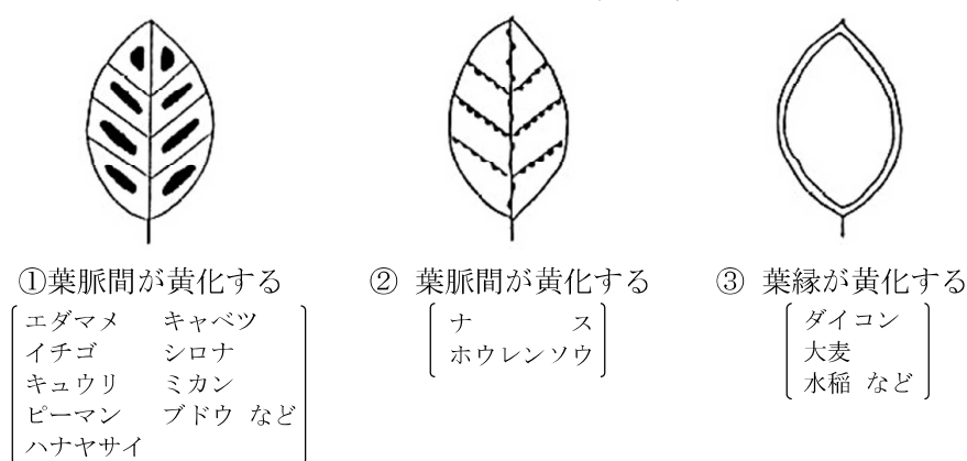
図3 マグネシウム欠乏症状の特徴
