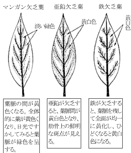
図4 欠乏症状の見分け方
