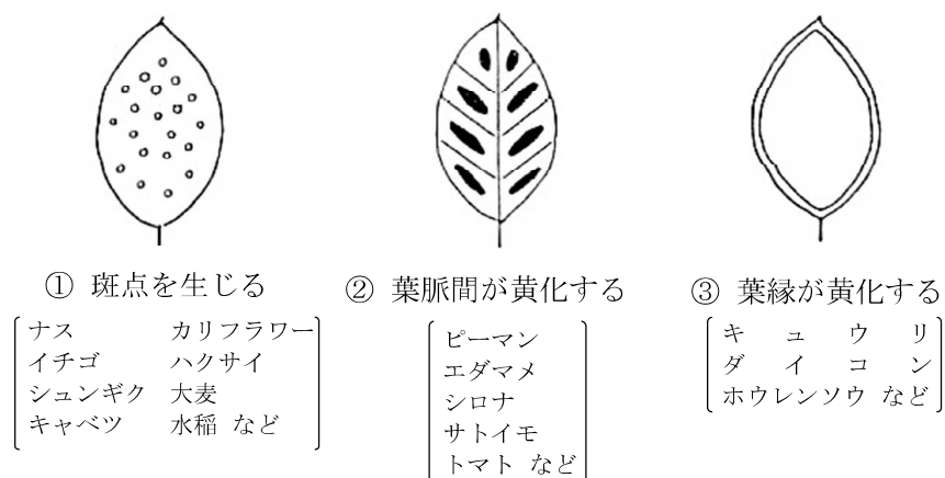
図2 カリウム欠乏症状の特徴
