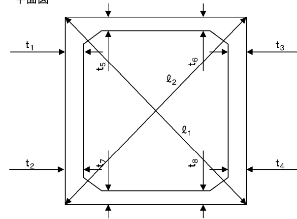
平面図
