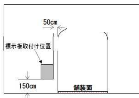
（取付図）
