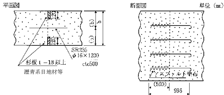
図 3-2 (収縮目地)
