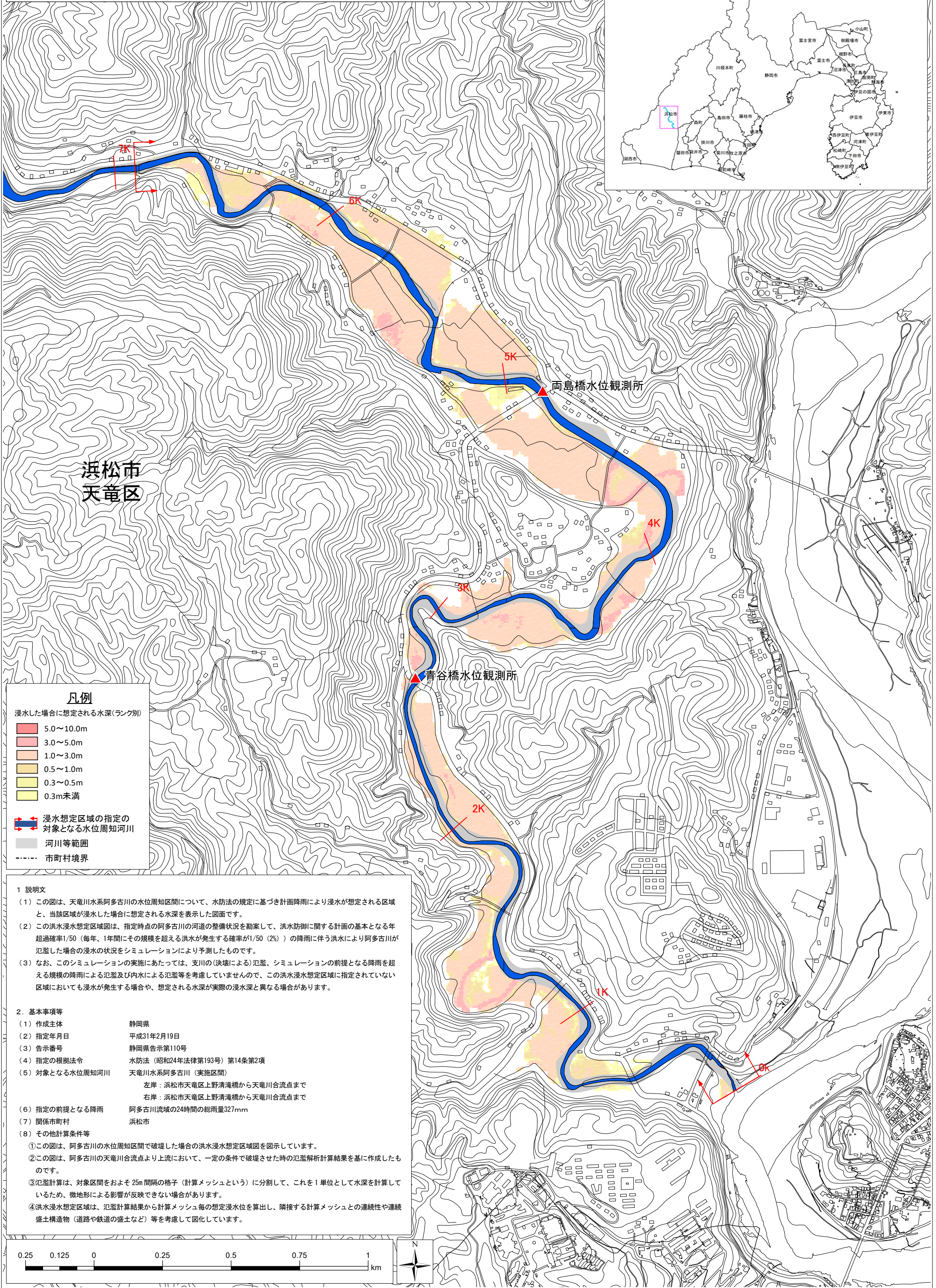
位置図
