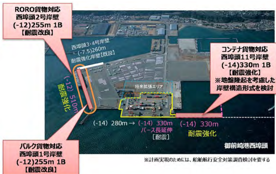
図 3-9 産業活動維持用の耐震強化岸壁の整備イメージ
