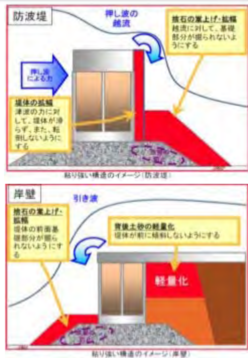
図3-4 防波堤のねばり強い構造への改良イメージ
