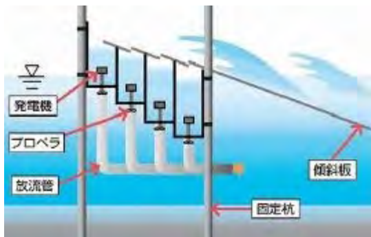
図4-13 越波型波力発電のイメージ
