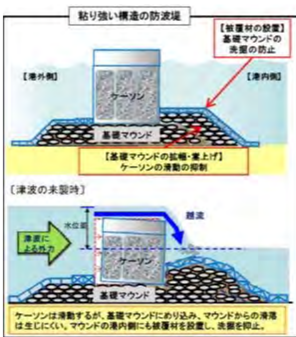
図3-4 防波堤のねばり強い構造への改良イメージ
