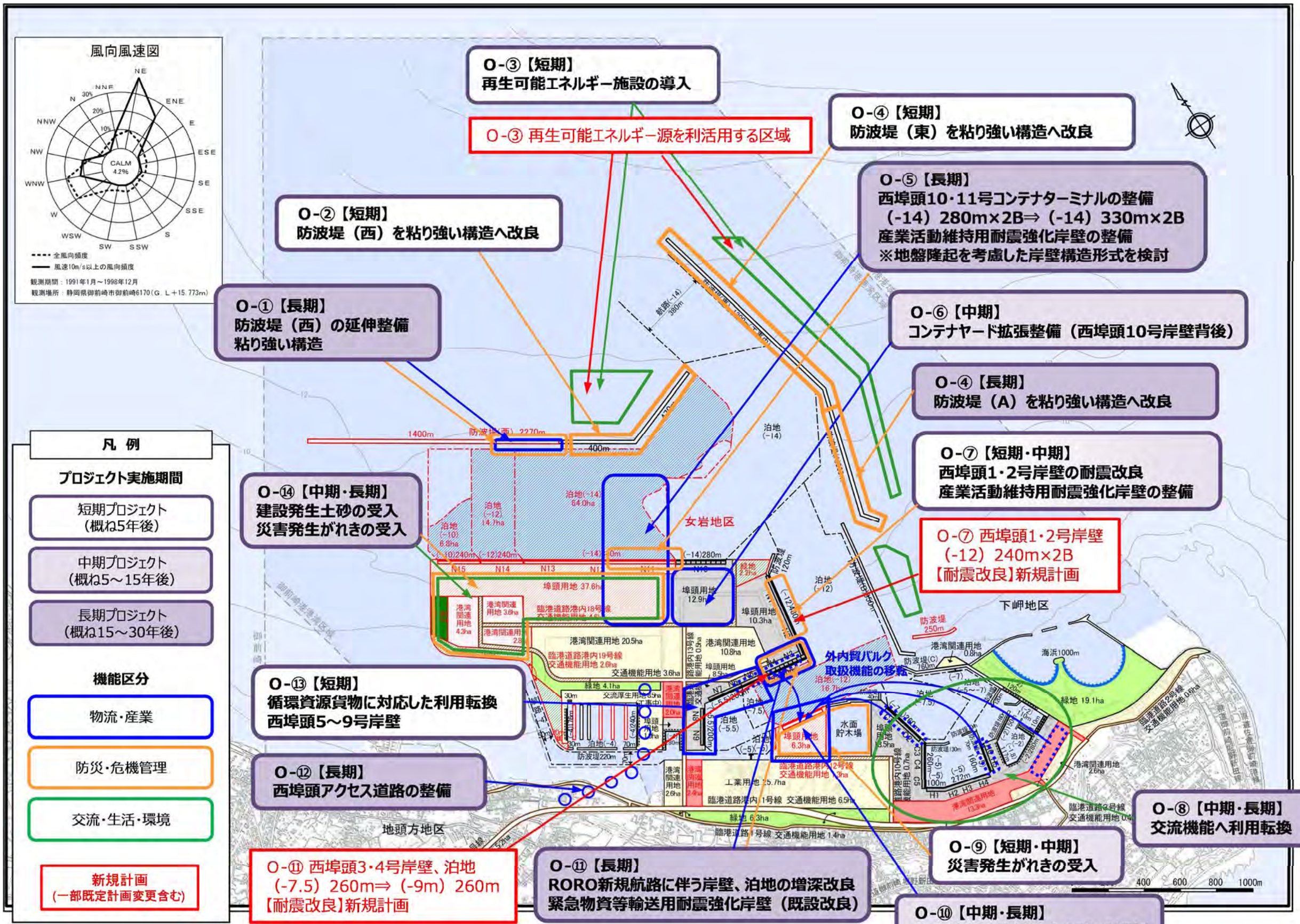
図 5-9 御前崎港の整備基本計画
