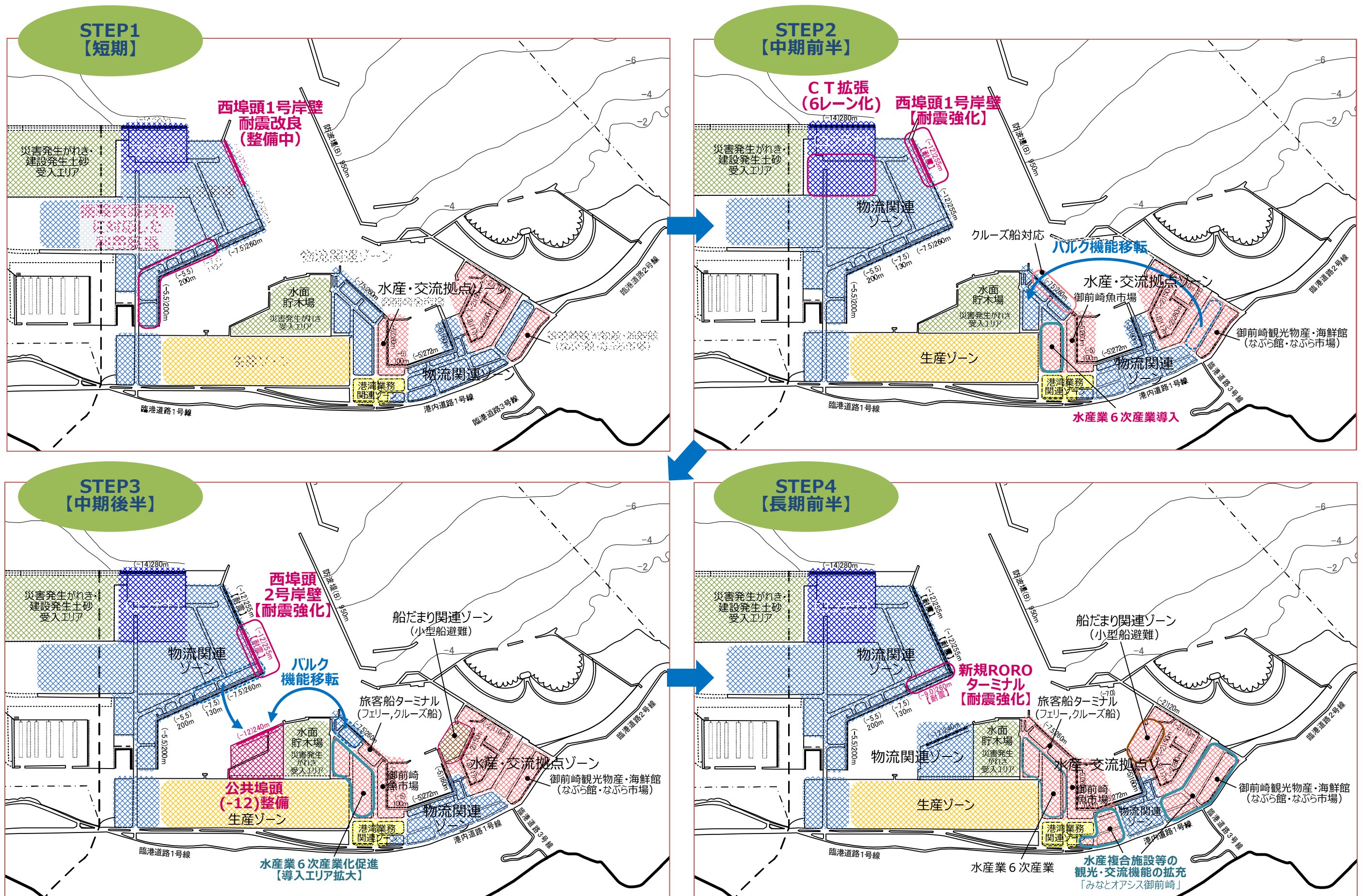
図 5-10 御前崎港の段階的機能再編イメージ (短期～長期前半)
