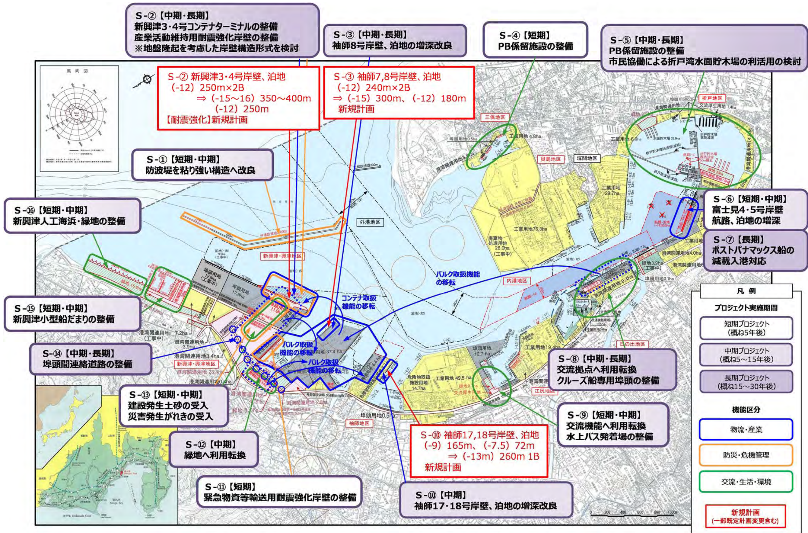
図 5-5 清水港の整備基本計画
