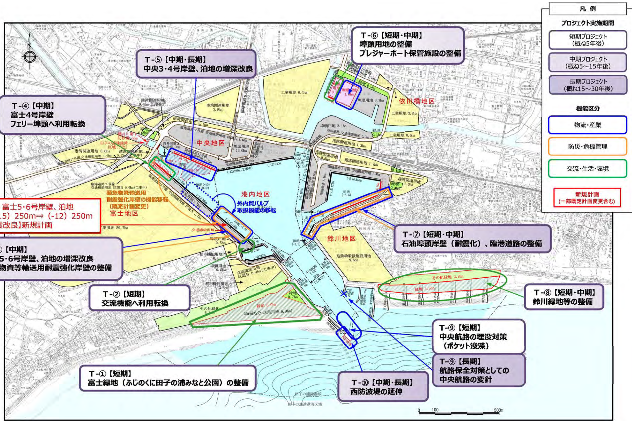
図 5-7 田子の浦港の整備基本計画
