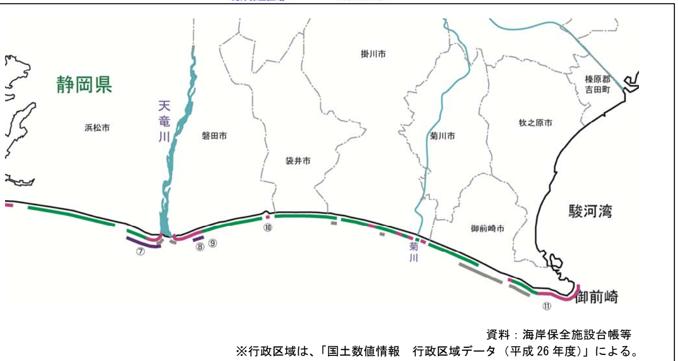
図 1.1.16 遠州灘沿岸の海岸保全施設の整備状況図
