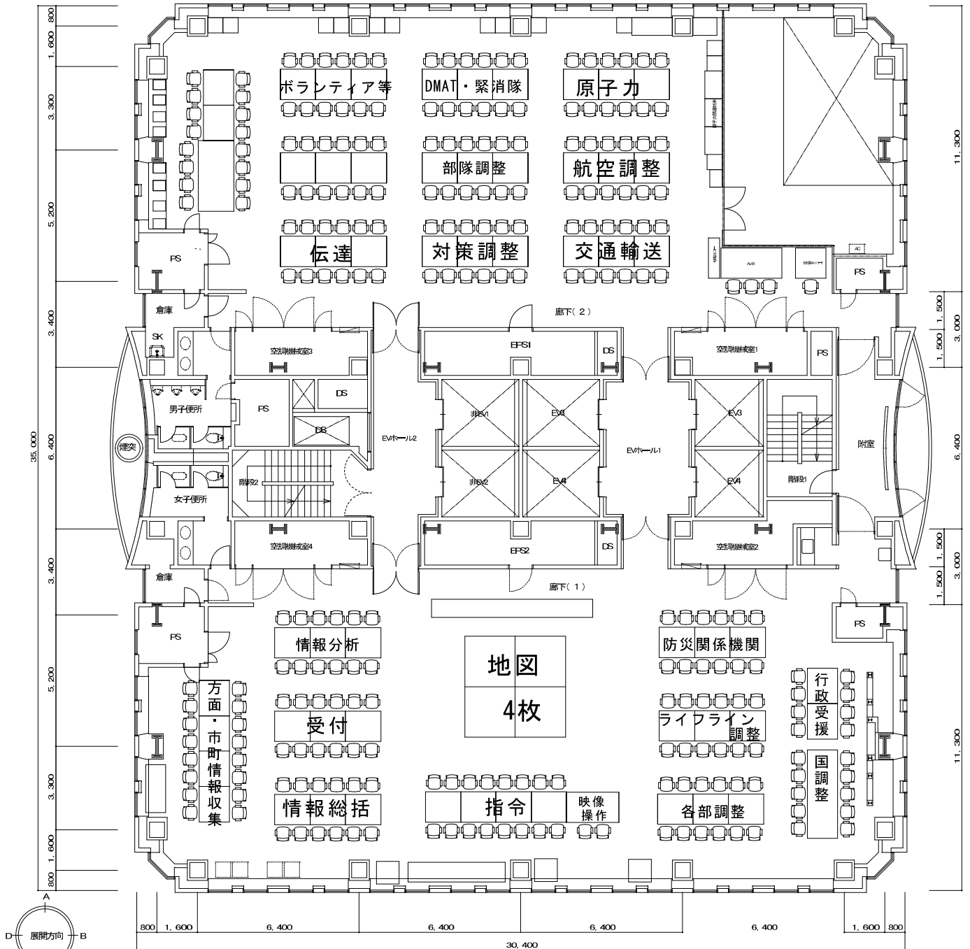
別館 5 階平面図
