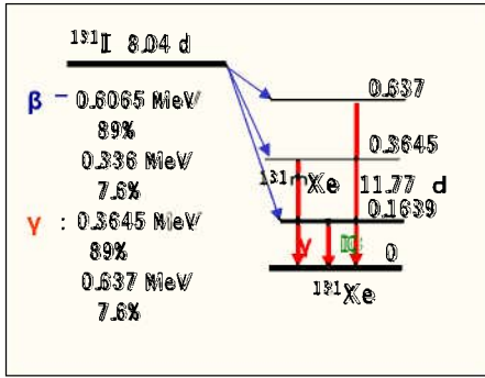
131 Iの壊変図
