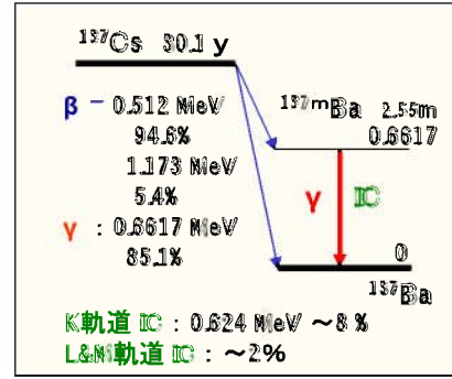
137 Csの壊変図
