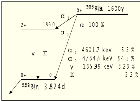
226 Raの壊変図
