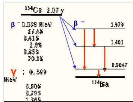
134 Csの壊変図
