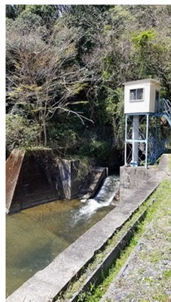
小水力発電の建設箇所
