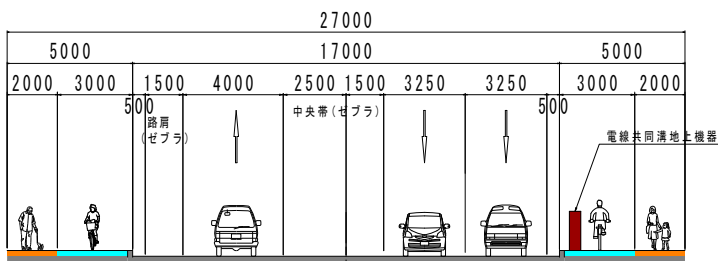
計画横断面図
