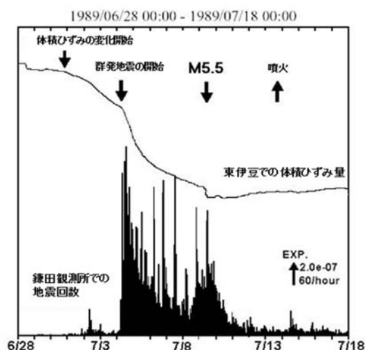
図 1.2.1 平成元年（1989年）噴火時の体積ひずみと地震回数の変化 （宮村ほか（2010）を一部改編）
