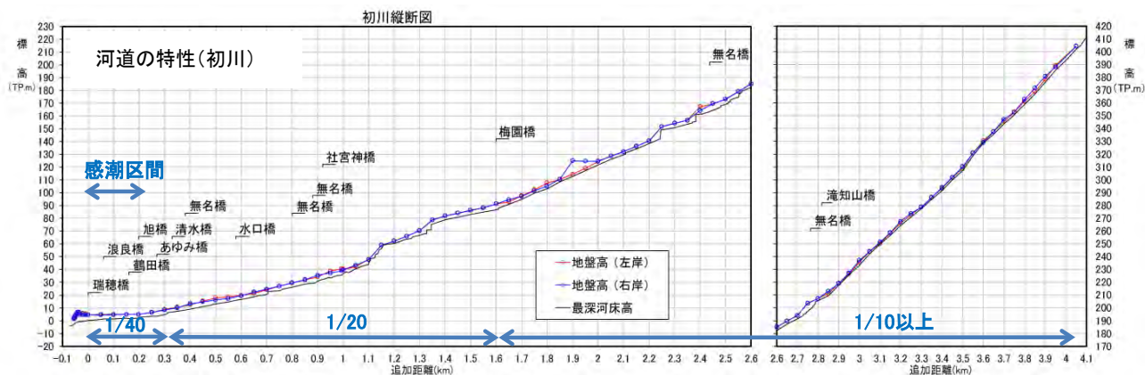
図 1-13 初川現況河道縦断面図
