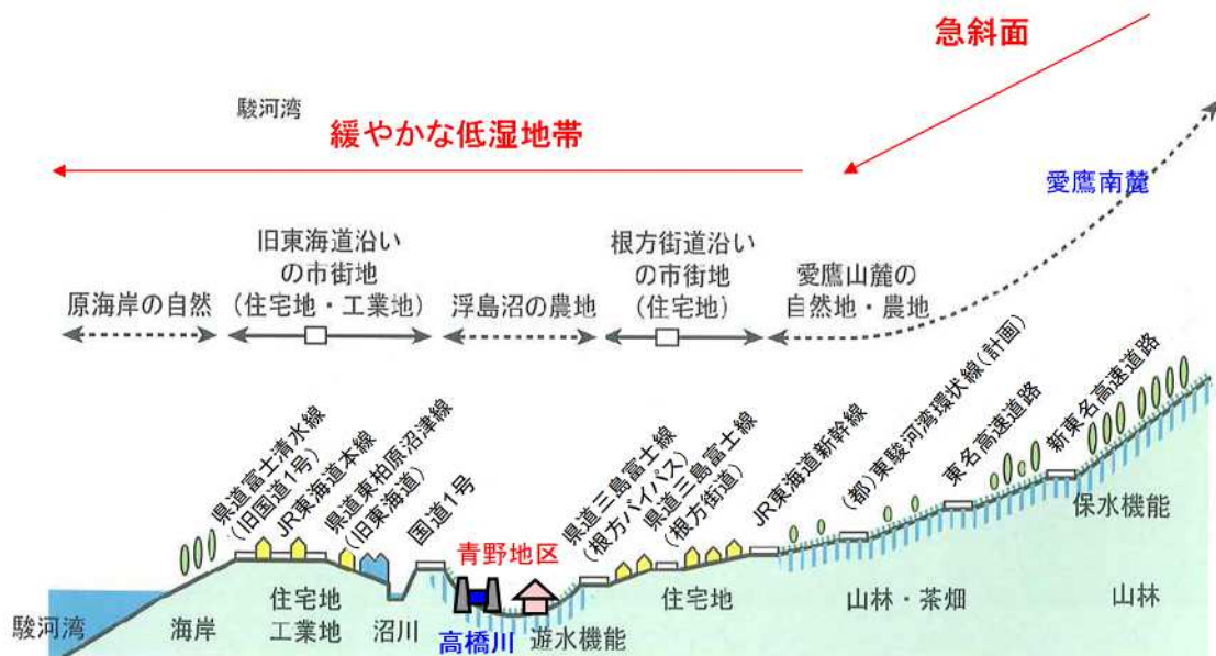
図 2-3 地形の特徴
