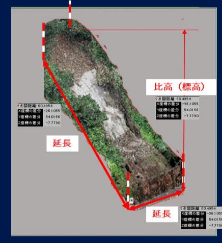
被災範囲抽出と形状寸法計測
