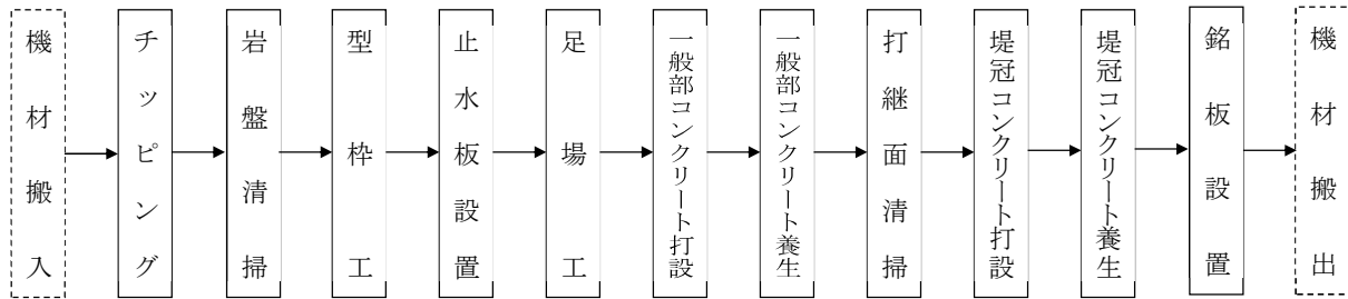
図2-1 施工フロー
