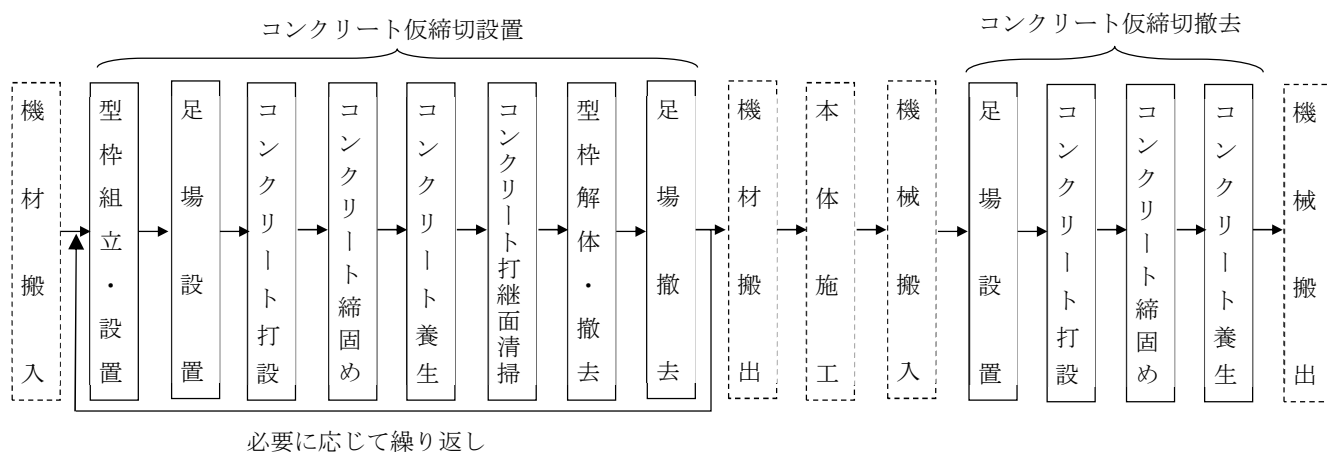
図2-1 施工フロー
