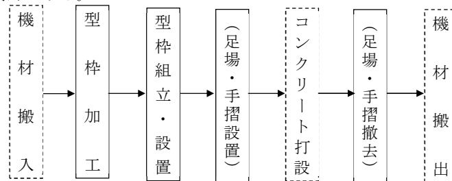
図 2-1 施工フロー
