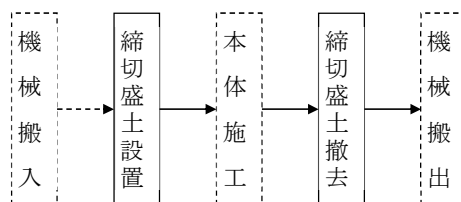
図 2-1 施工フロー
