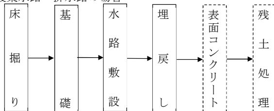
図2ー1 施工フロー
