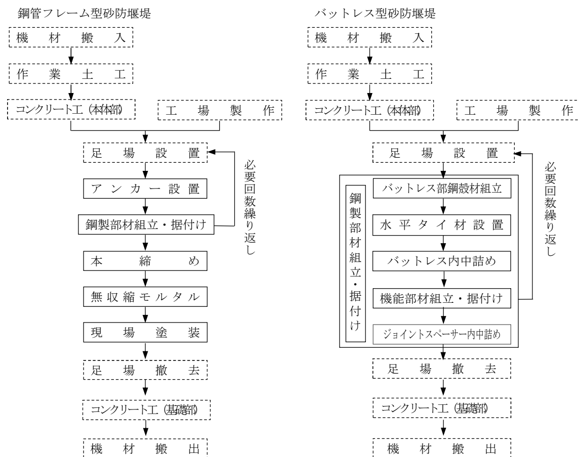
図2-1 施工フロー
