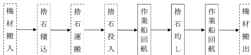
図2-1 施工フロー
